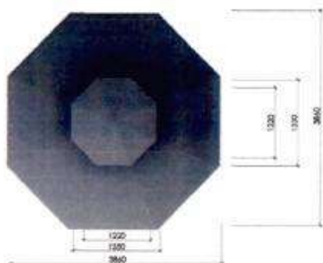
Типовой внешний вид киоска № 2
